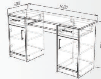
Тумба під ТВ 140 TV-stand 140
