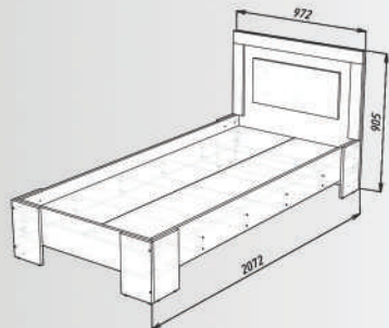
Ліжко (відкрите) 90 Bed (open) 90
