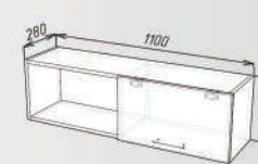
Стіл 2П/ Desk 2Sh
